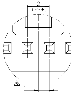
詳細図1 Scale 10:1
