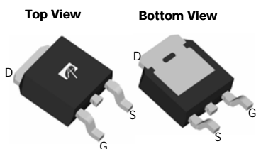
TO252 DPAK
