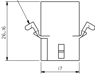
MT'G EARS (表参照) 参照 DETAIL A OR B
