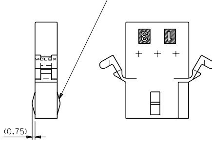
LOCKING TAB (表参照)
