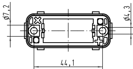
Montageausschnitt/ 1:1 panel cut out
