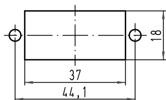
Montageausschnitt/ 1:1 panel cut out
