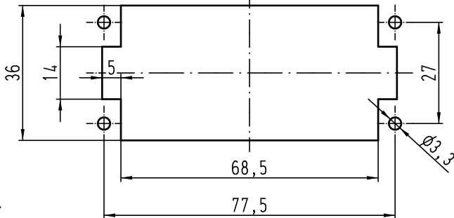
Montageausschnitt panel cut out
