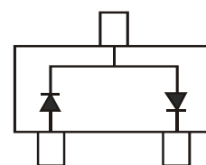
BAT54SW-KL8
