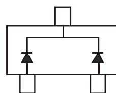
BAT54CW-KL7
