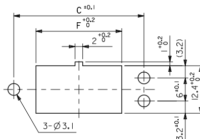
パネル切抜寸法 (参考)
