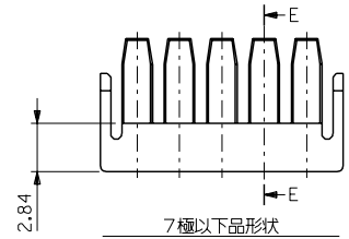
7 極以下品形状 SHAPE OF UNDER 7 CKT.
