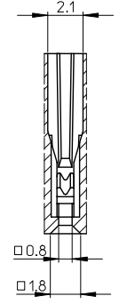
断面 K-K SECTION K-K
