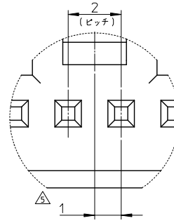
詳細図1 Scale 10:1
