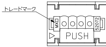
13極から17極の形状 (カバーの形状のみ異なる)
