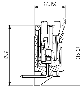
嵌合断面図
