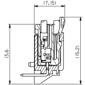
嵌合断面図
