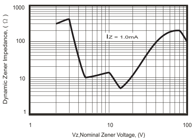
Fig.3- Zener Voltage vs Zener Impedance
