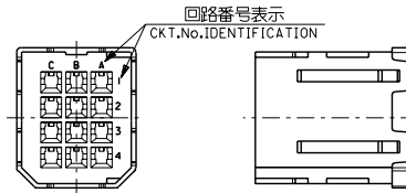
電線挿入側 WIRE SIDE
