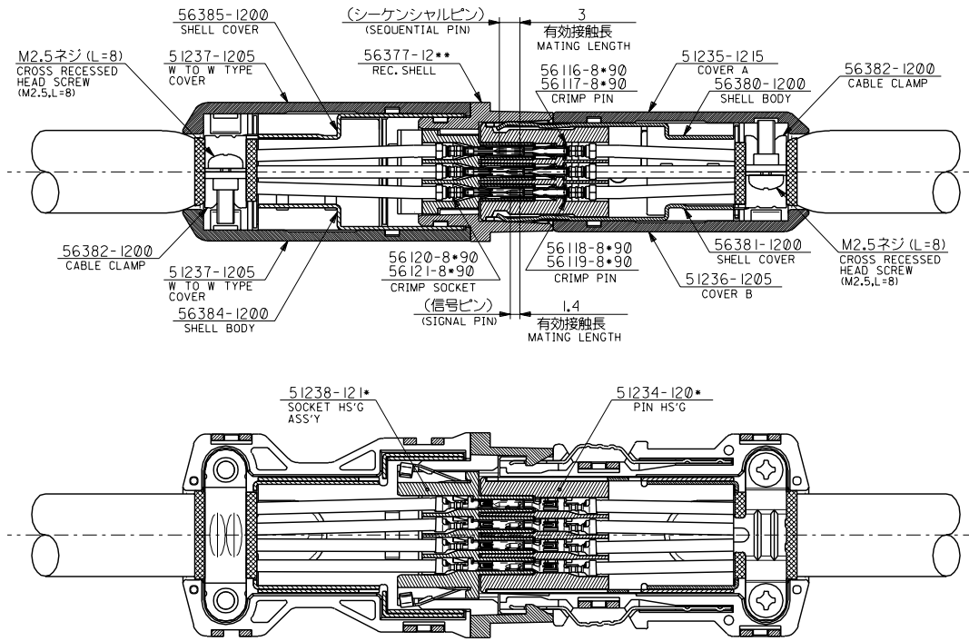
嵌合図 (中継タイプ)
