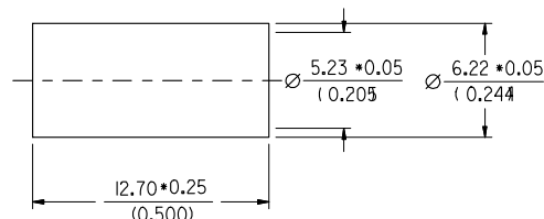
FERRULE
