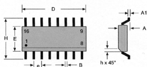
HMC1022—16-Pin SOIC
