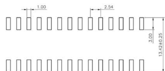
P.C.B LAYOUT
