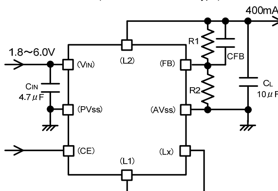
Circuit (XCL208F/XCL209F Type)
