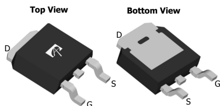
TO252 DPAK
