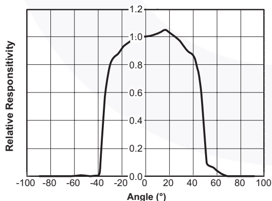
Fig. 1 Normalized Reception Pattern for the ALS Detector
