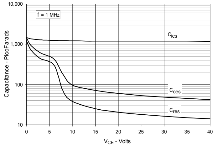
Fig. 10. Capacitance
