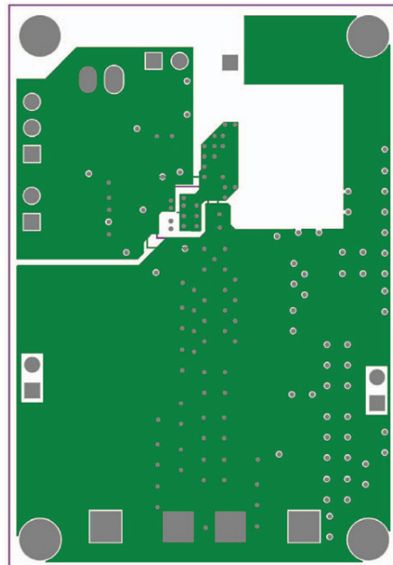
Fig. 22 - Inner Layer 2
