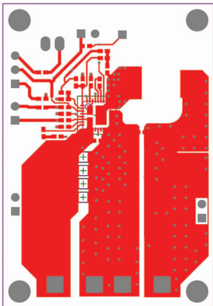
Fig. 20 - Top Layer
