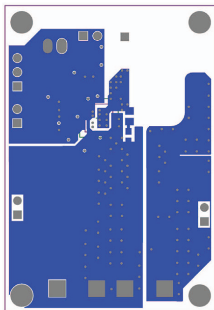
Fig. 23 - Bottom Layer
