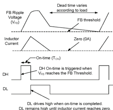
Fig. 6 - Power-Save Mode
