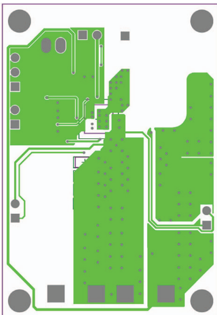
Fig. 21 - Inner Layer 1
