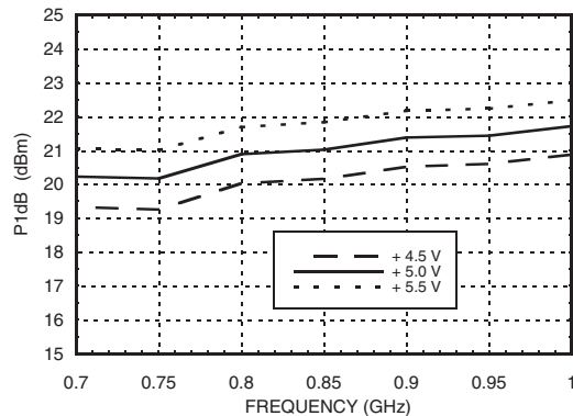
P1dB vs. Vdd
