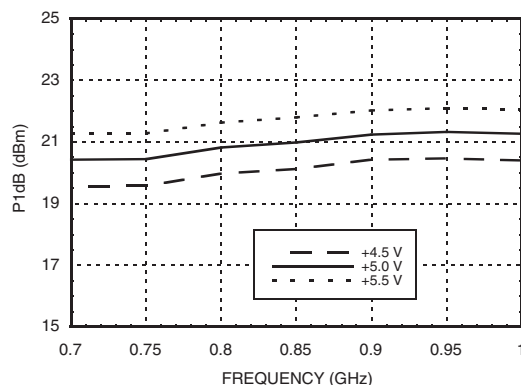
LNA P1dB vs. Vdd
