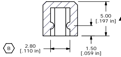
SECTION A-A SCALE 4 : 1
