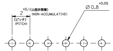
基板取付穴推奨寸法
