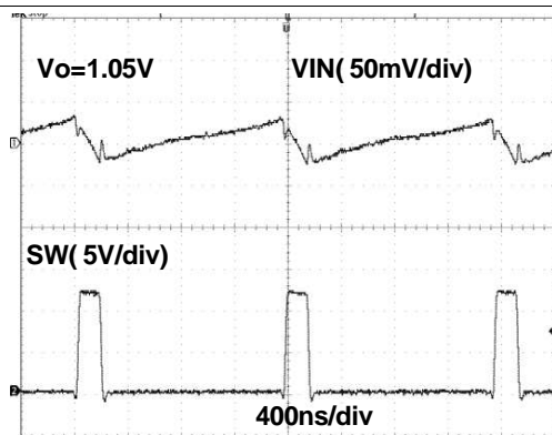
Figure 15. VIN Ripple
