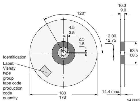
Fig. 11 - Reel Dimensions - GS08
