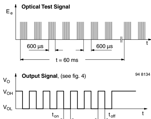
Fig. 3 - Output Function
