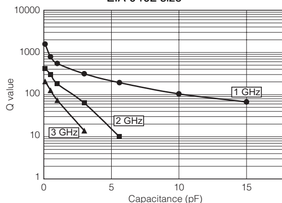
EIA 0402 size
