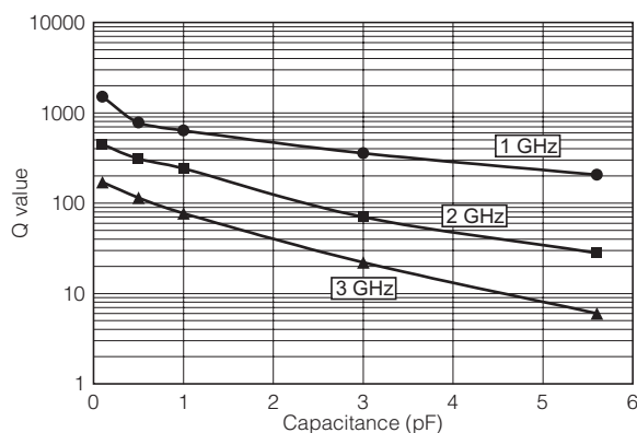
EIA 0201 size
