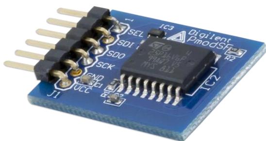
The PmodSF.
