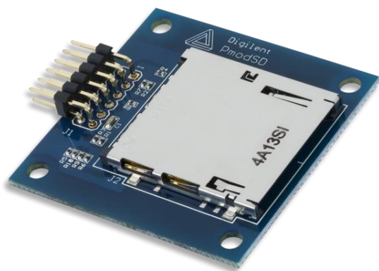
The PmodSD.
