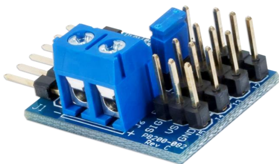
The PmodCON3.
