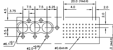
LAY-OUT PCB - HOLE
