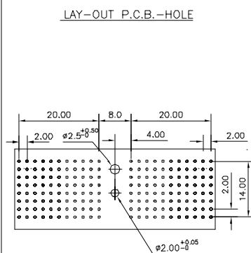
LAY-OUT P.C.B.-HOLE
