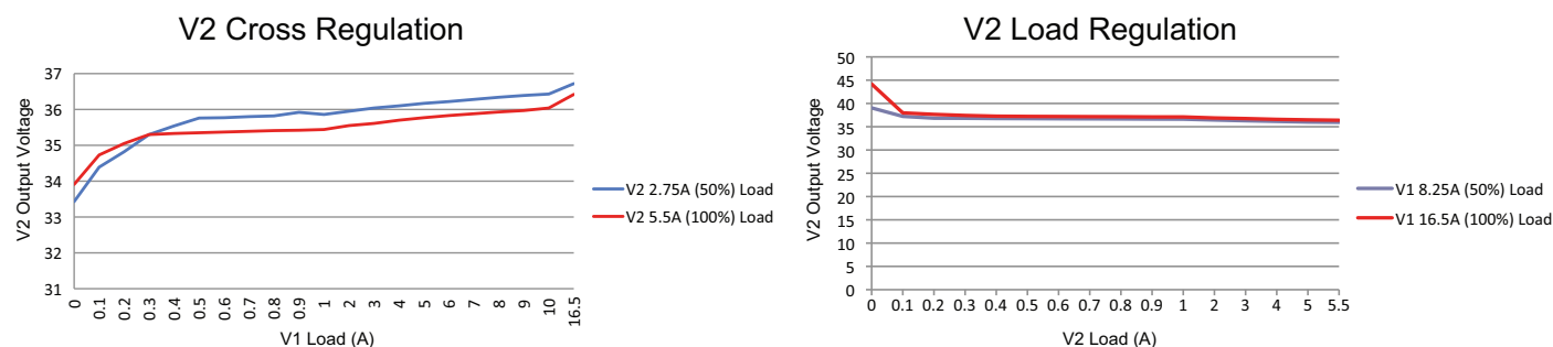
Figure 3 - EMH350PD22
