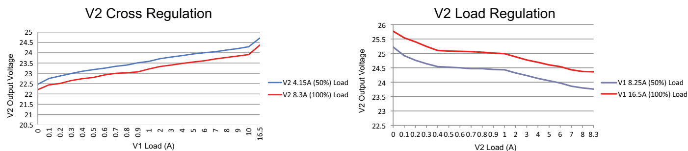
Figure 3 - EMH350PD22
