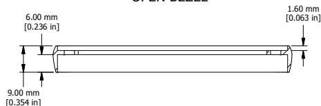
OPEN BEZEL
