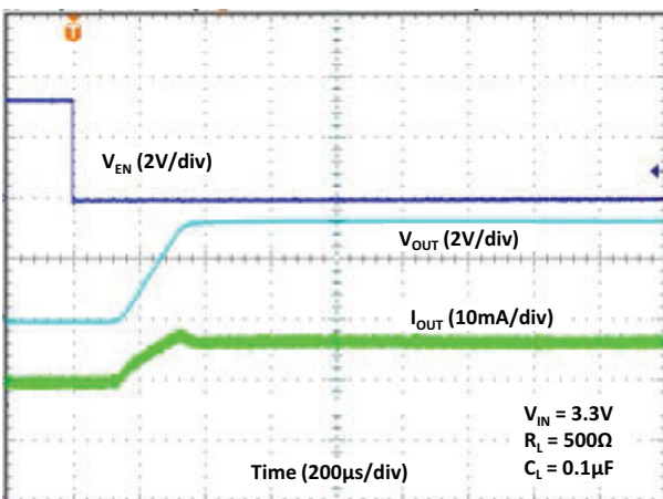
Fig. 24 - Turn-on Time
