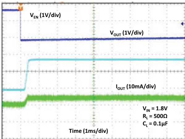
Fig. 23 - Turn-on Time
