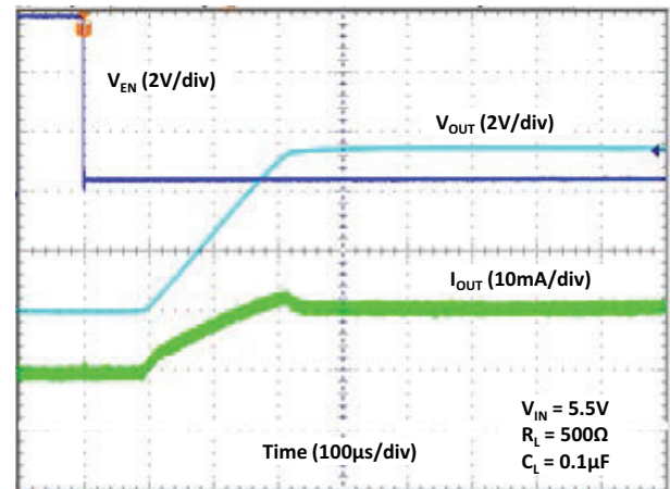
Fig. 26 - Turn-on Time
