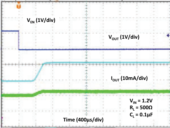
Fig. 22 - Turn-on Time
