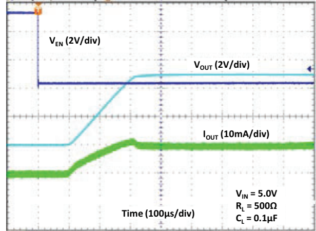
Fig. 25 - Turn-on Time
