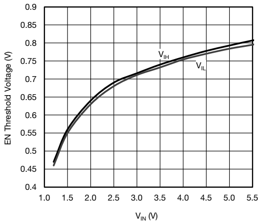
Fig. 17 - EN Threshold Voltage vs. Input Voltage
