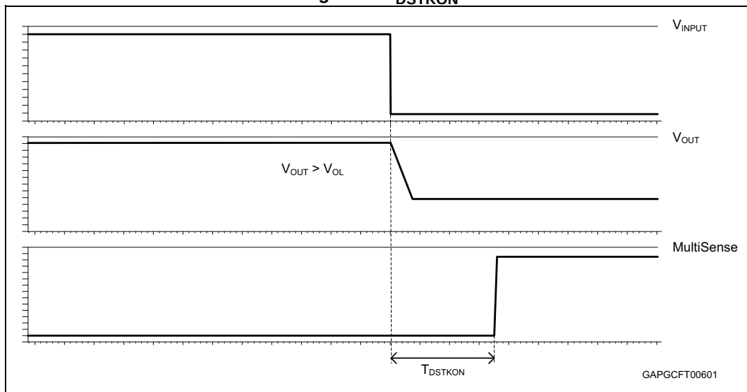
Figure 9. T_{DSTKON}
