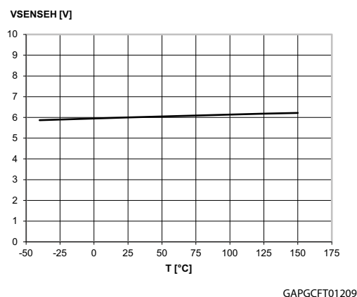
Figure 34. V_{\text{senseh}} vs. T_{\text{case}}
