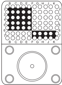
71W1 70 #22
