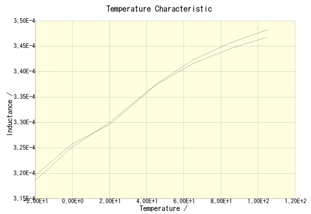
CLF10040T-331M-CA(DC = 0A)
