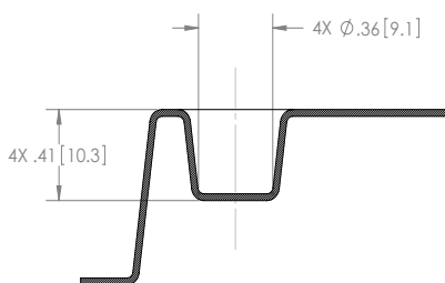
SECTION D-D SCALE 2:1
