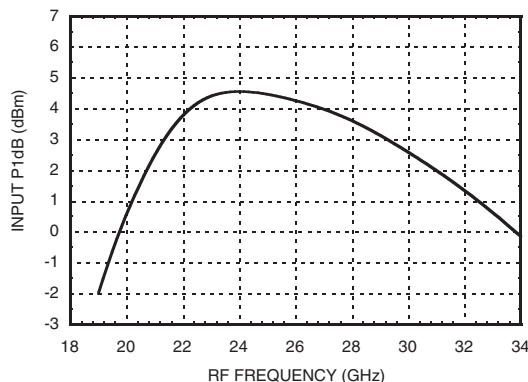
Input P1dB @ LO = -4 dBm, Vdd = +4V
