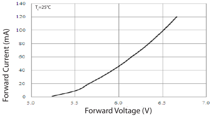
V_f ----- I_f
