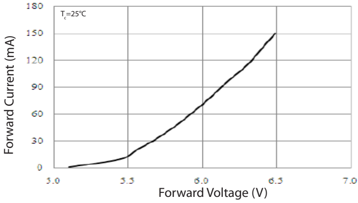
V_f ----- I_f
