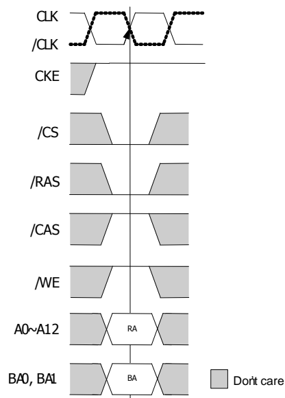
Figure11 : Active command
