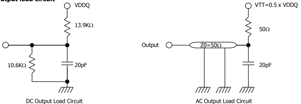
Figure10 : Output load circuit
