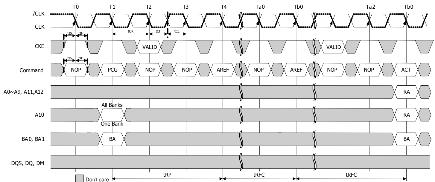
Figure34 : Auto refresh
