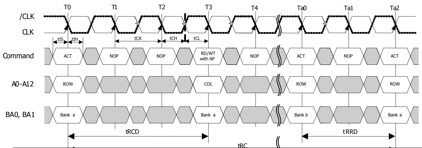
Figure12 : tRCD, tRRD, tRC
