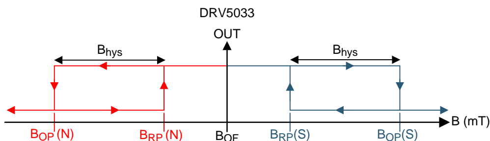
Figure 12. DRV5033— B_{OP} > 0
