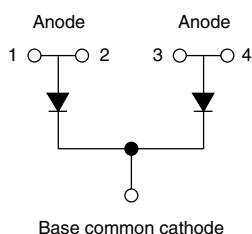
SOT-227
